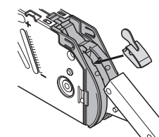
SCHEMA MONTAGGIO LIMITATORE LIMITER INSTALLATION DIAGRAM
